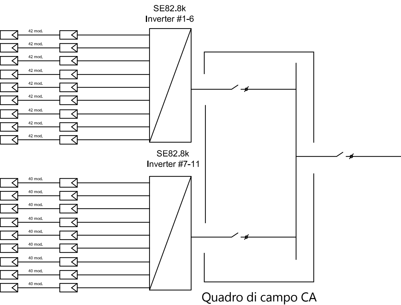
Soluzione di inverter ottimizzato CC SolarEdge
